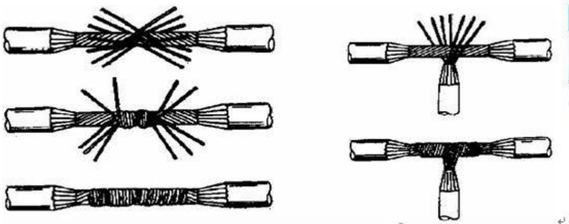
◀图 2> 多股线常见接头接法▶
