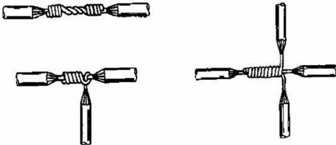
◀图 1> 单股线常见接头接法▶
